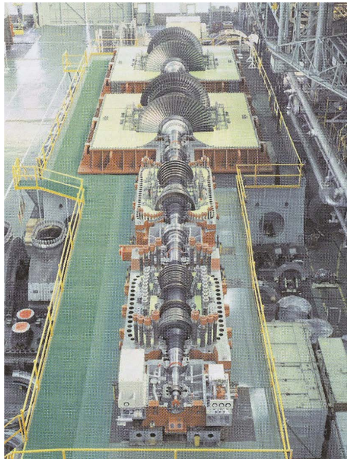
写真27 中部電力碧南3号700MWタービン工場組立 [提供] 三菱重工業(株)
