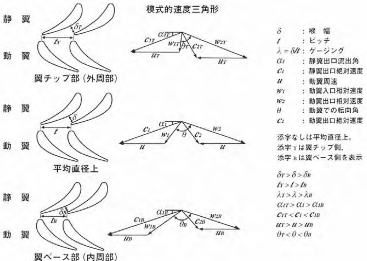
図 41 平行翼の翼高さ方向の状態変化
